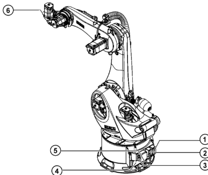
Fig. 6-9: Interfaces A1 to A6
